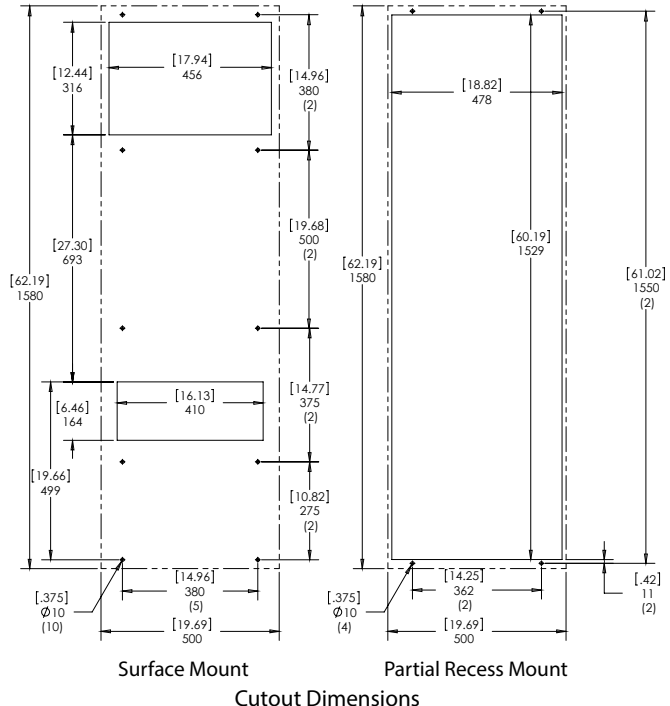
Cutout Dimensions
